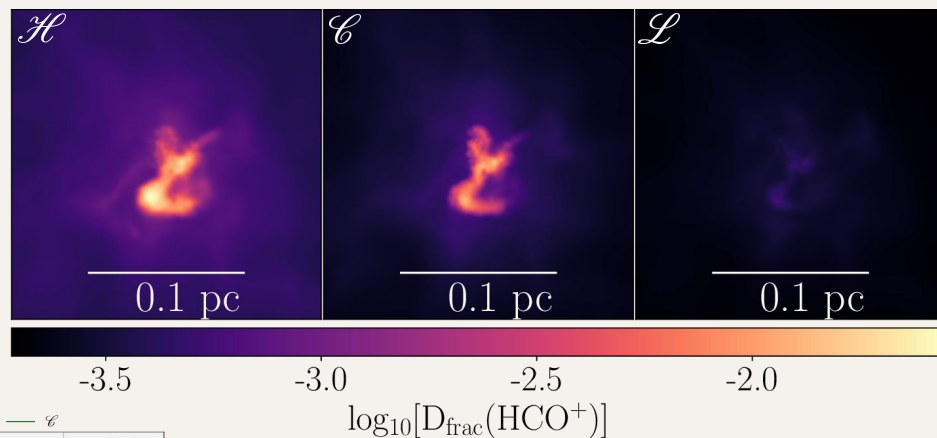
Fig. 3: Deuteration of \text{HCO}^+ .
